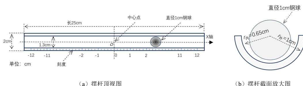
图 3 摆杆结构示意图
